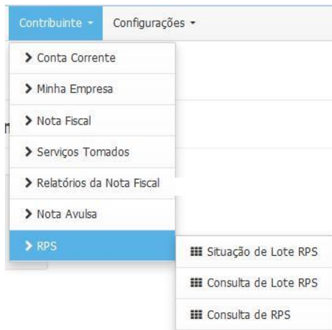
Figura 75 – Menu RPS
